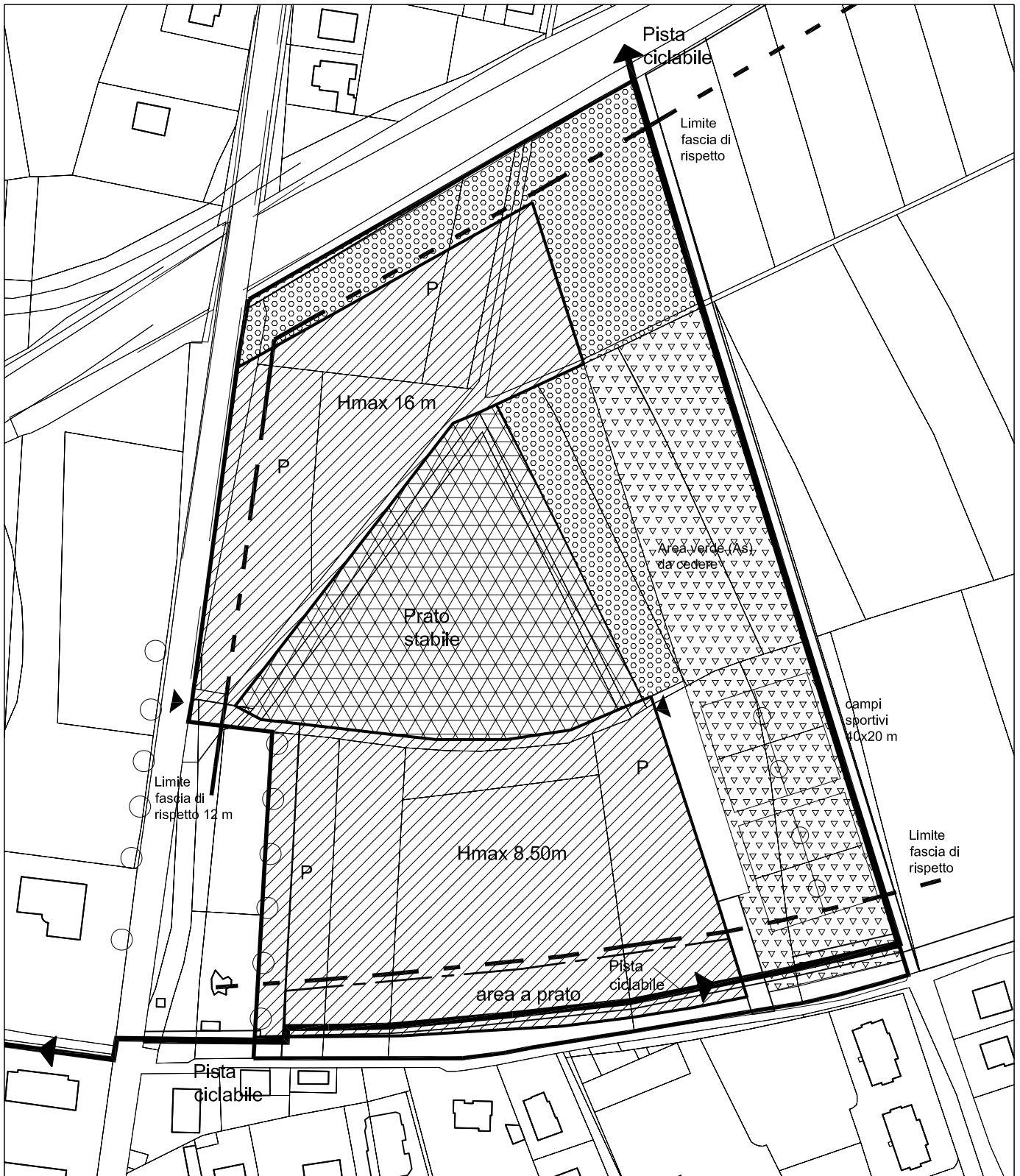
Estratto planimetrico 1:2000
