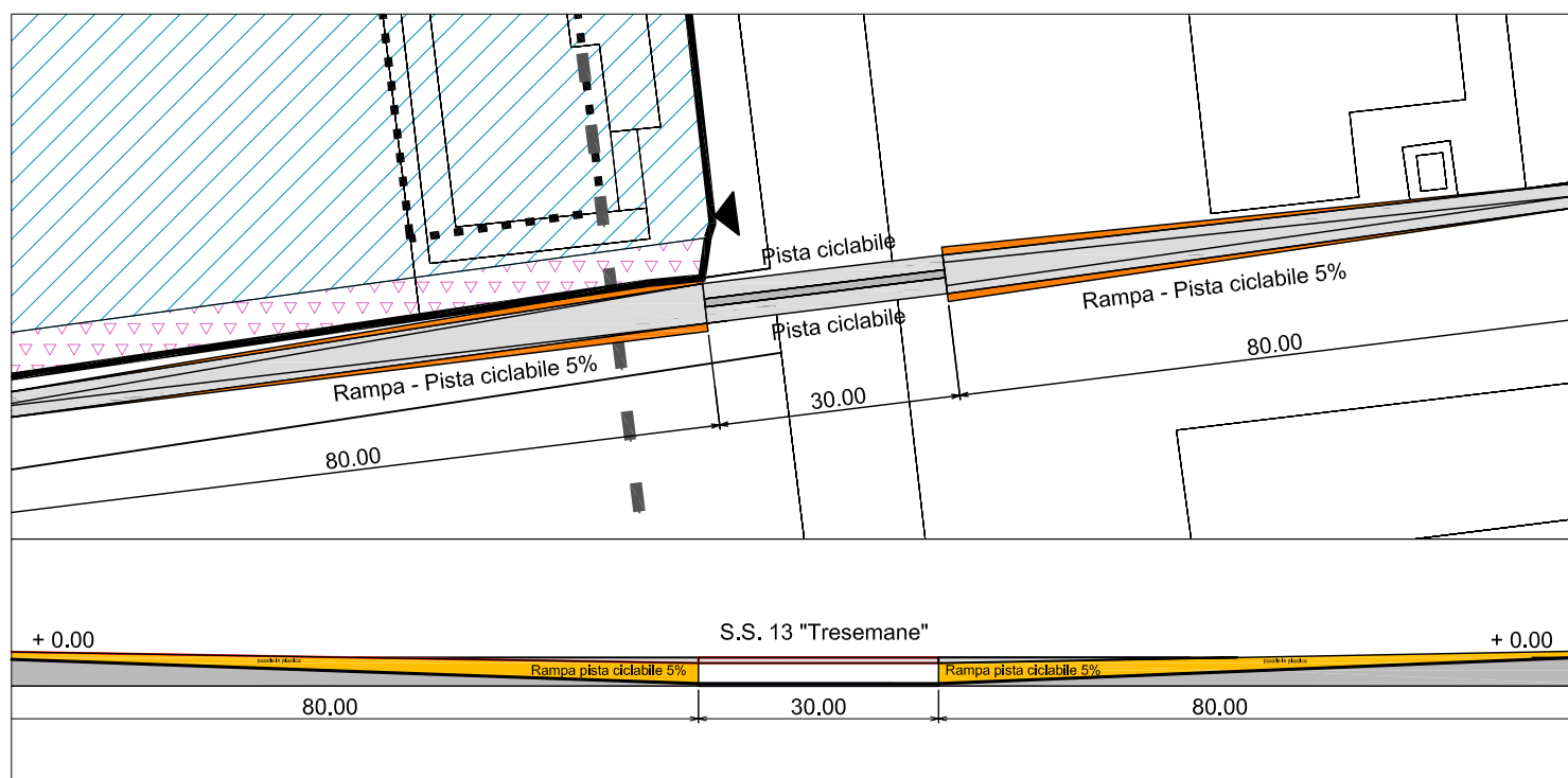
Ipotesi sottopasso 1:1000
